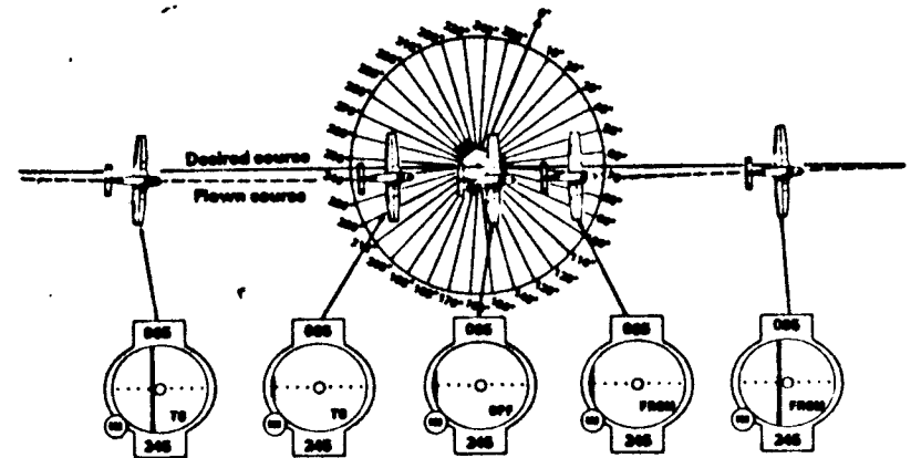
Figure 14. VOR Passage
