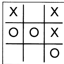
Fig. 11.10: Move 3
