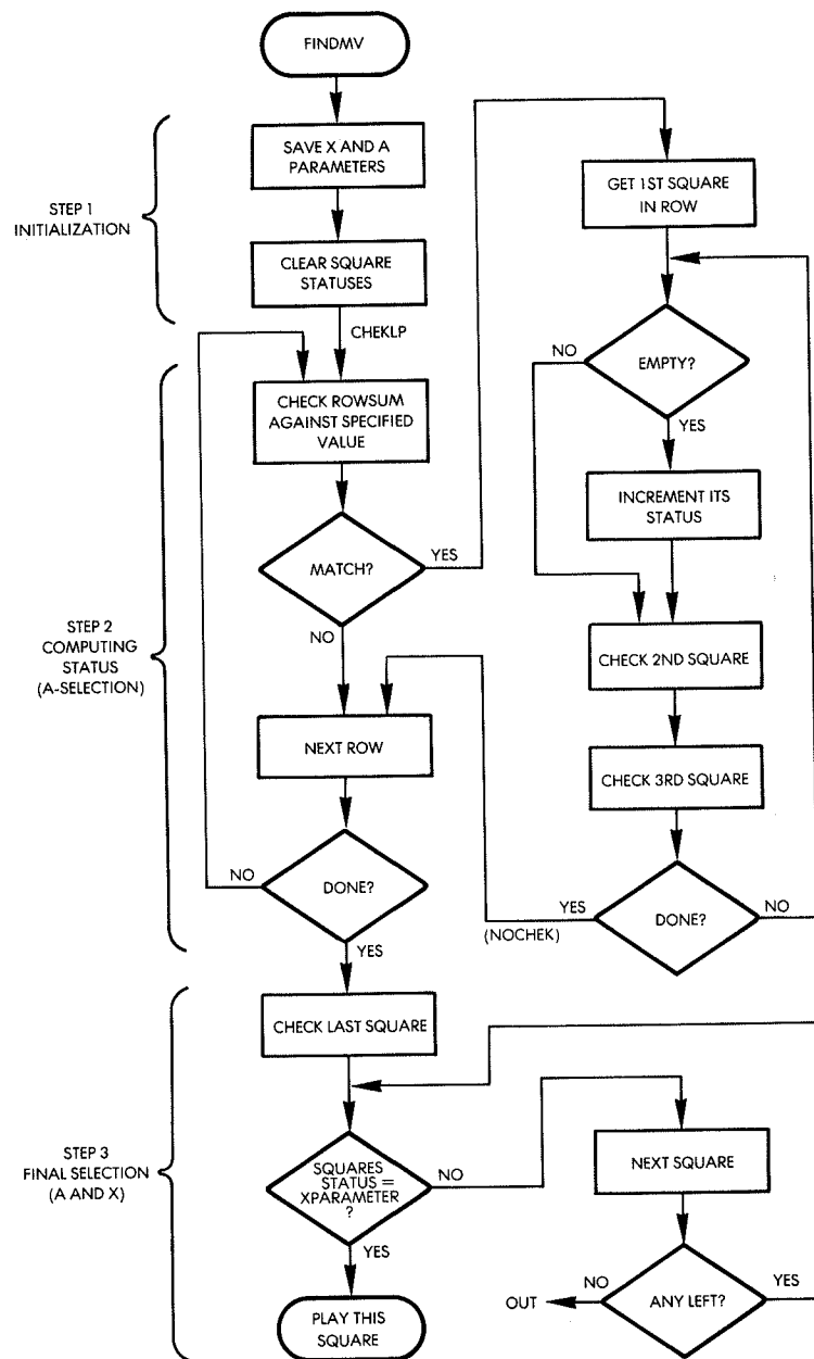
Fig. 11.49: FINDMV Flowchart
