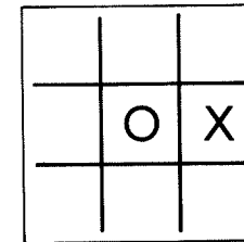
Fig. 11.12: Move 1
