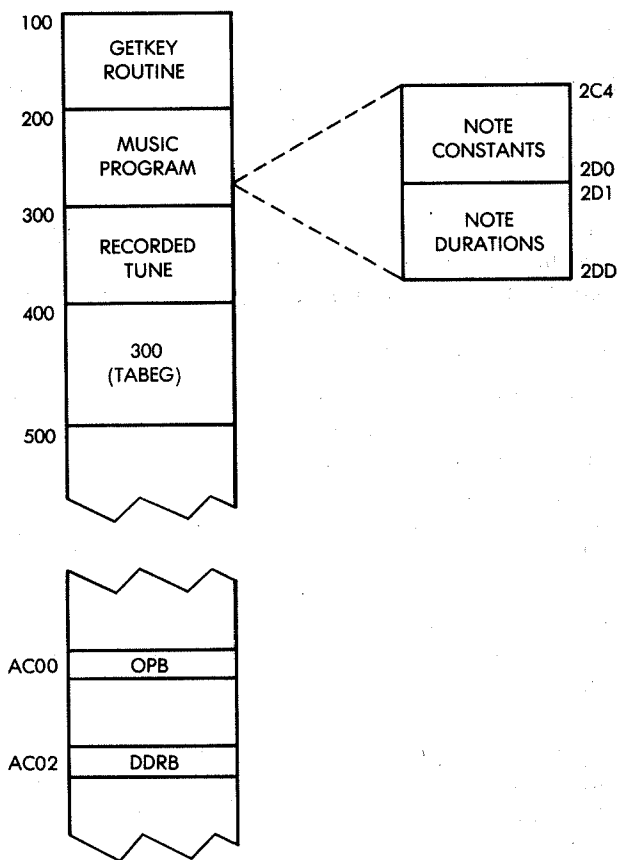
Fig. 2.4: Memory Map
