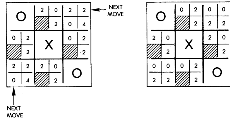
Fig. 11.35: Trap 3
