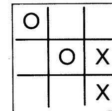
Fig. 11.13: Move 2
